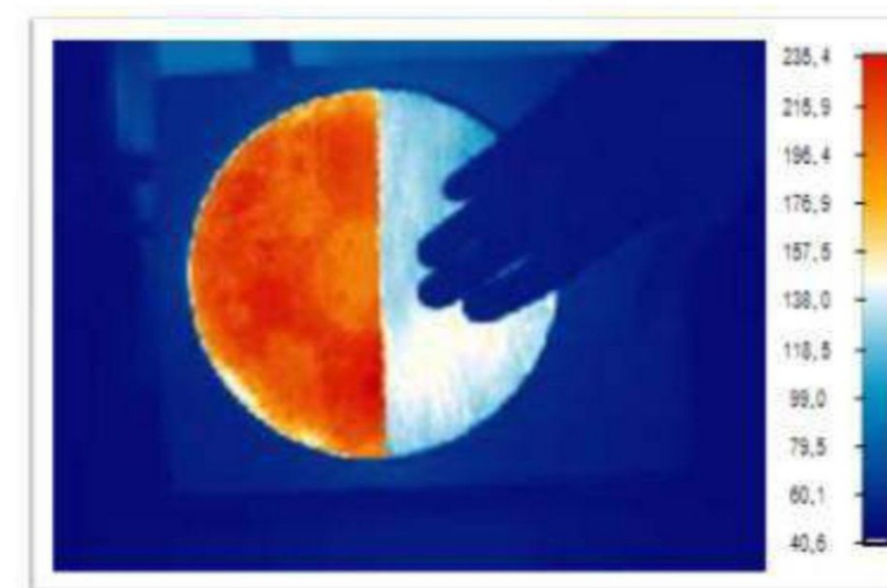
СЪЕМКА ЭЛЕКТРОПЛИТЫ ТЕПЛОВИЗОРОМ, С ПОЛОВИНОЙ, ПОКРЫТОЙ ТЕПЛОИЗОЛЯЦИЕЙ БРОНЯ
